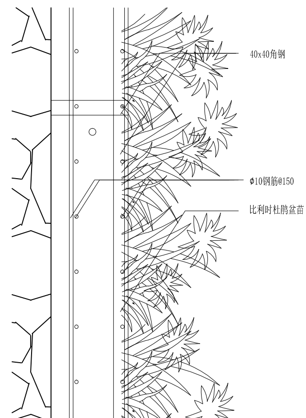
⑥ 植物墙大样2 1:30
