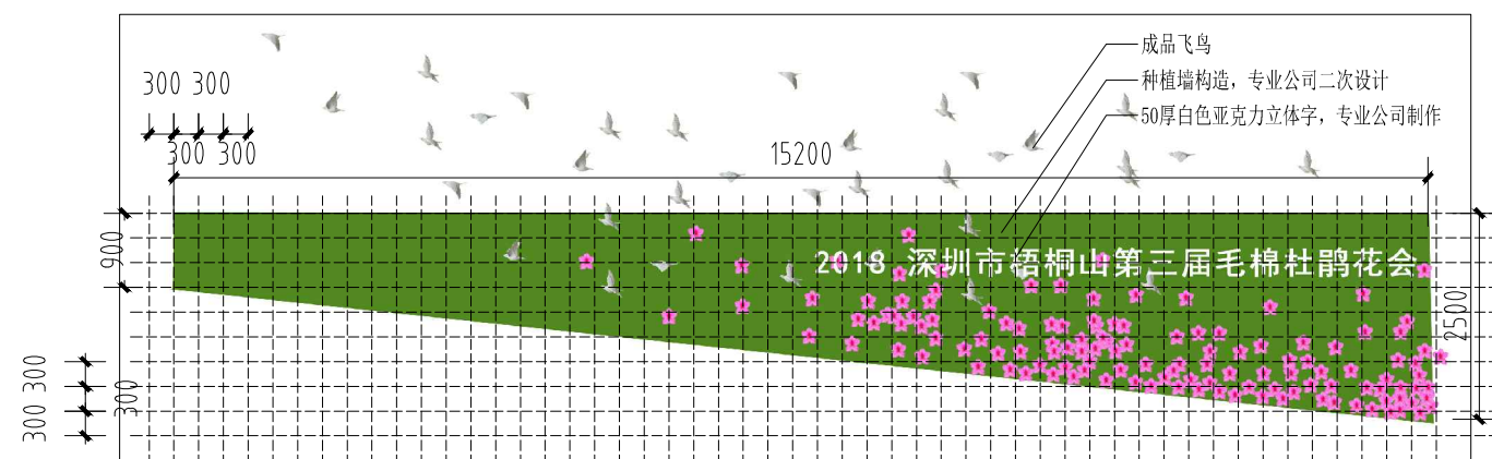
④ 入口挡土墙立面装饰 1: 100
