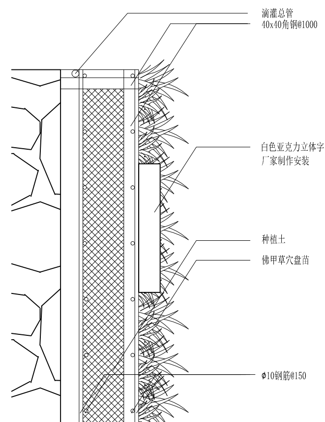
⑤ 植物墙大样1 1:30
