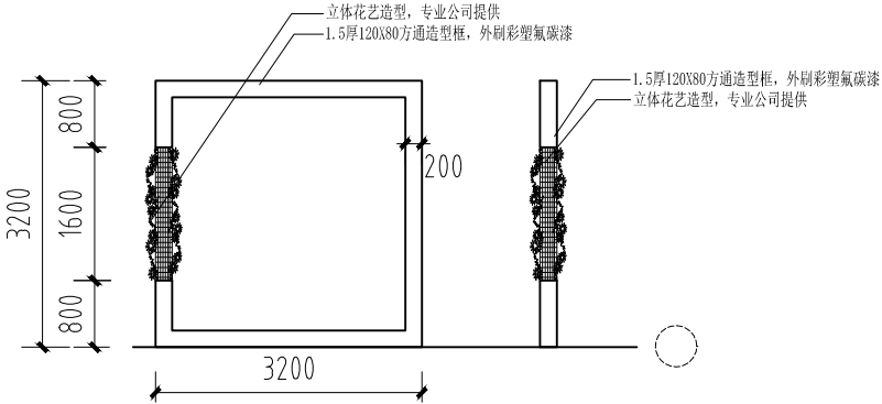
2 彩虹廊架单体 1: 100
