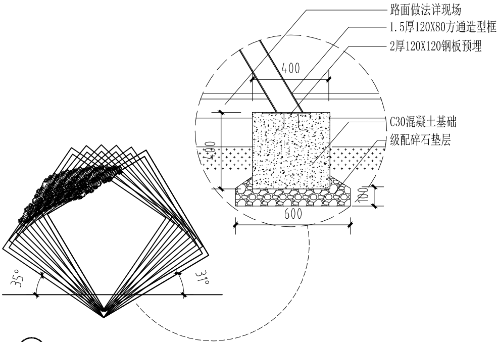
3 彩虹廊架立面图 1: 100
