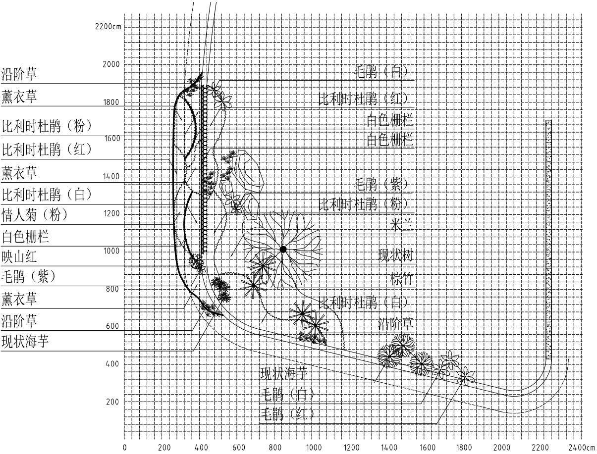
1 凤栖梧桐植物布置平面图 1: 200
