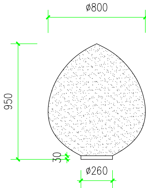
大号灯罩：壁厚4.0mm
